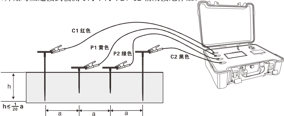
接线示意图
