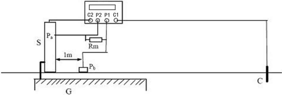
接触电压、接触电位差测试接线示意图
