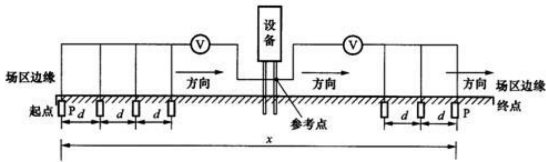
图 6 场区地表电位梯度分布测试示意图 P—电位极；d—测试间距。
