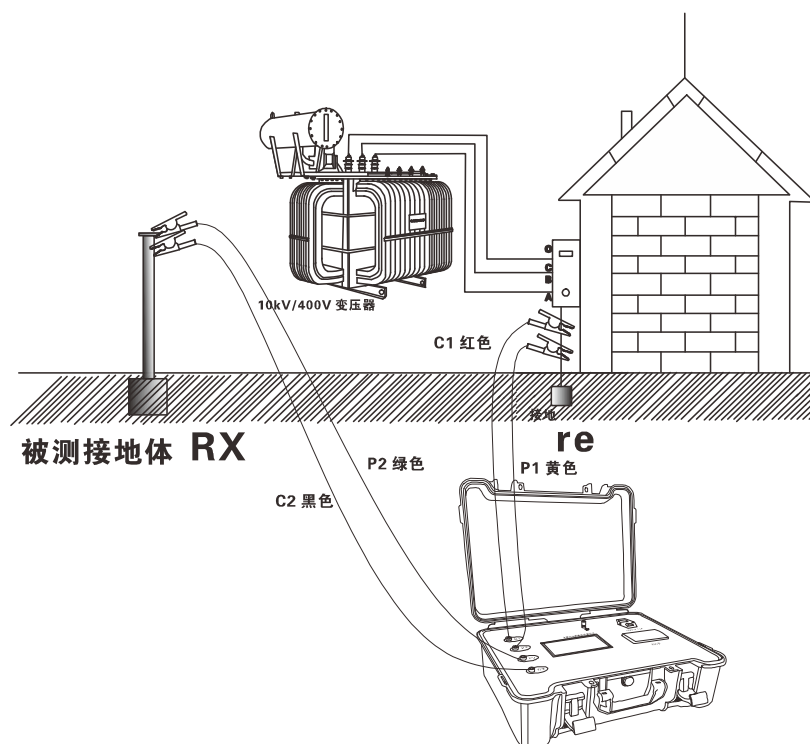
图 3.1 回路阻抗法测试杆塔接地阻抗接线示意图
