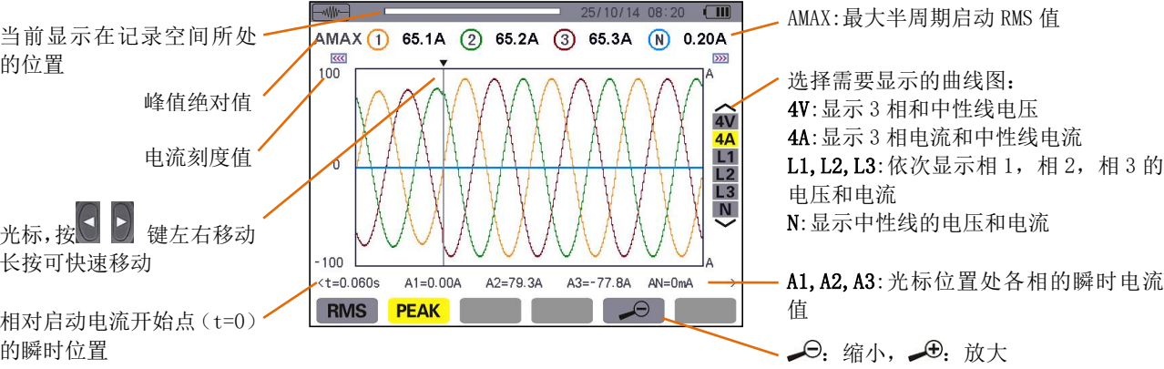
图 6-11 4A 峰值显示屏幕
