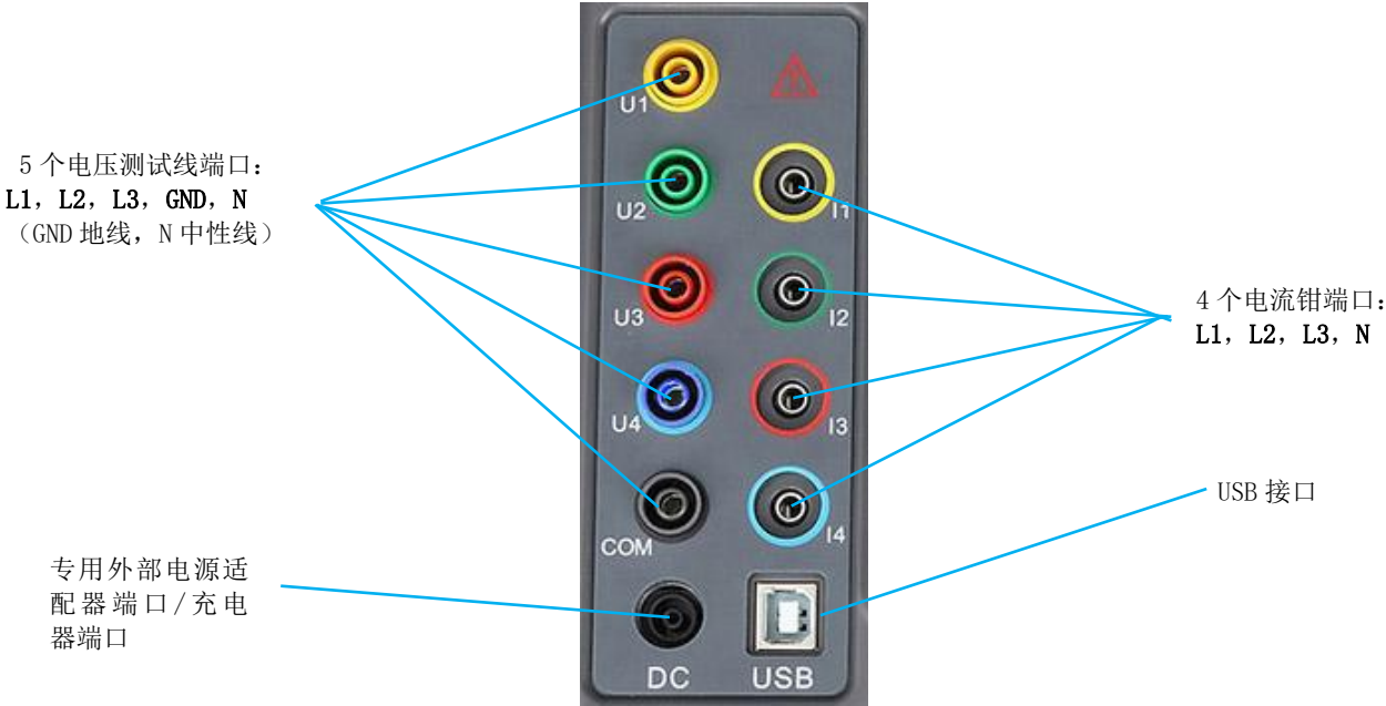
图 3-3 接口面板
