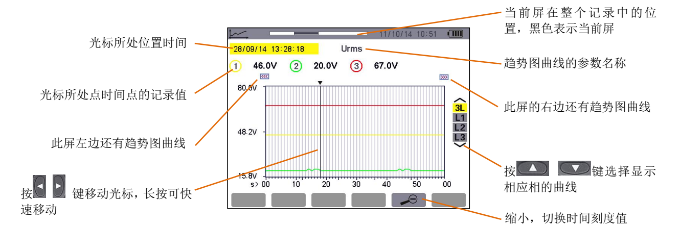
图 10-10 线电压有效值不包括最大、最小、平均值
