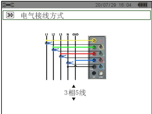
图 4-7 三相 5 线连接
