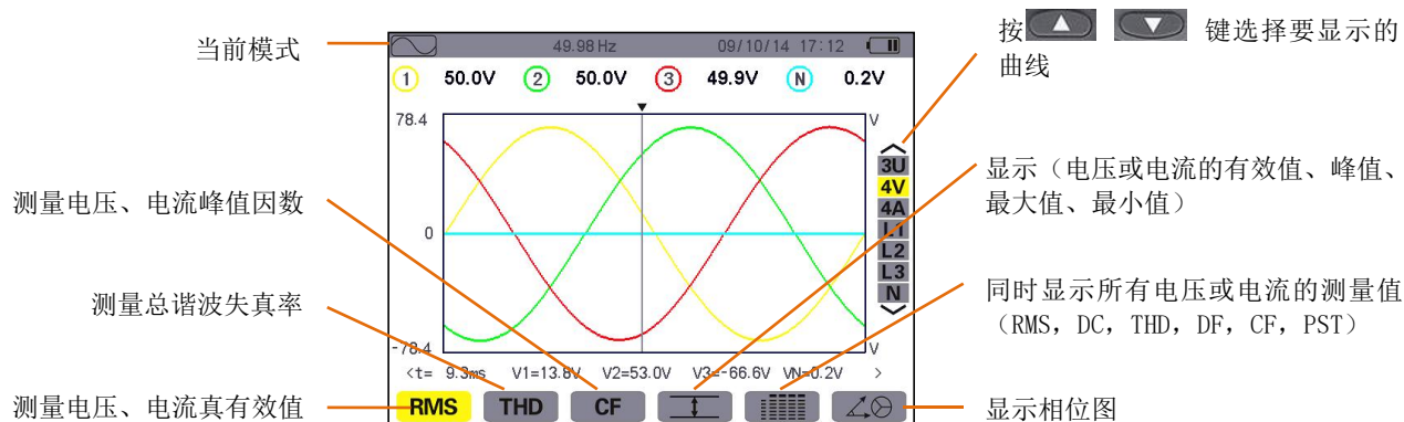
图 8-1 波形模式屏幕
