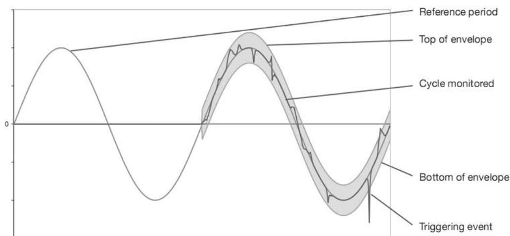
图 17-4 暂态捕捉触发原理图解
