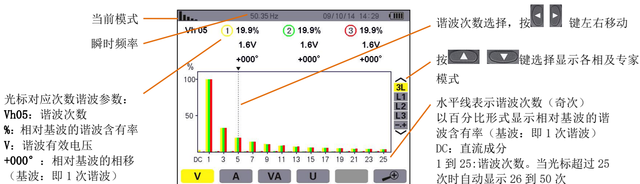
图 7-2 相电压谐波 3L 显示
