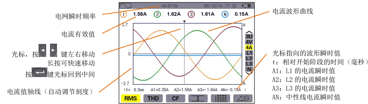
图 8-4 4A 下 RMS 显示屏幕
