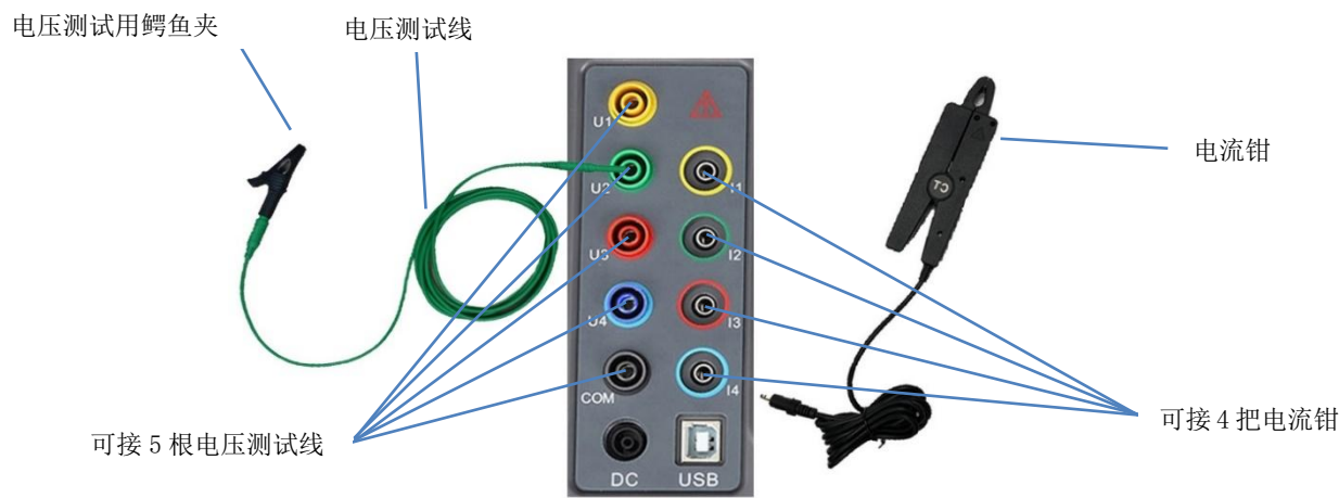
图 4-3 顶端测试连接
