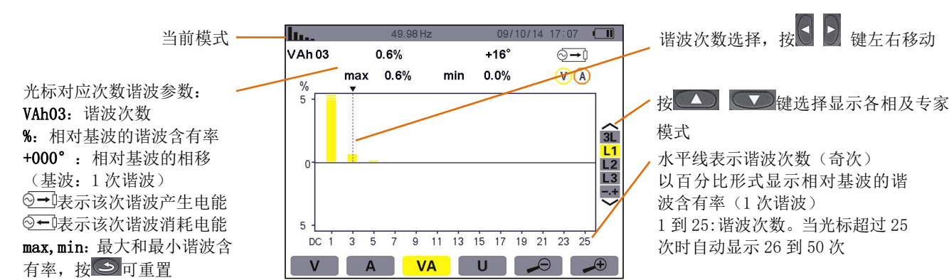
图 7-7 视在功率谐波 L1 显示
