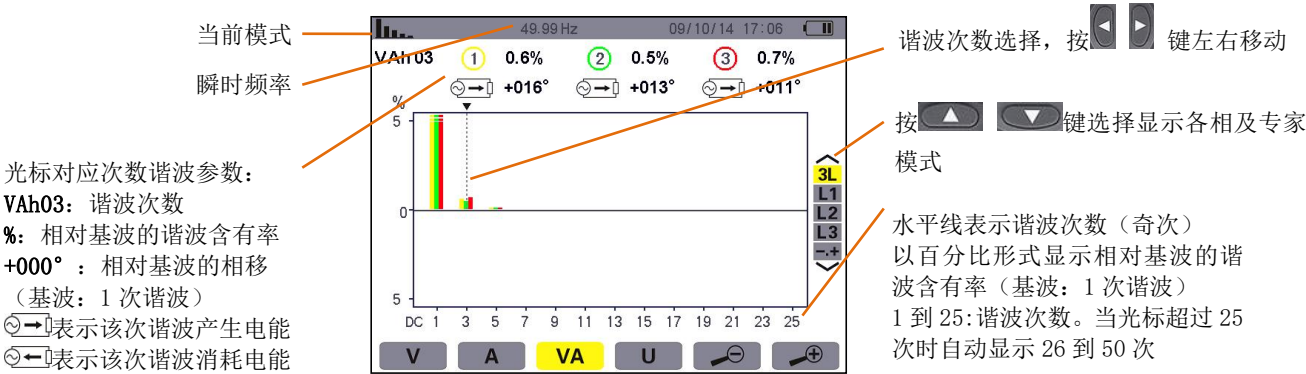
图 7-6 视在功率谐波 3L 显示
