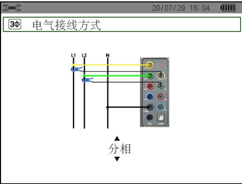
图 4-5 分相连接
