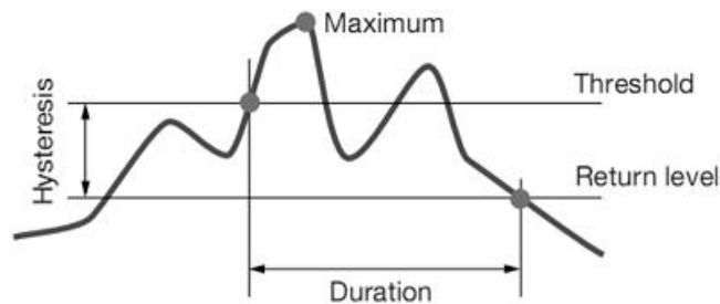
图 17-1 骤升侦测回差图例
