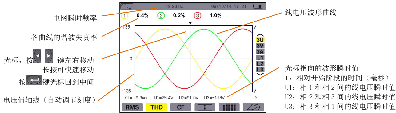
图 8-6 3U 下 THD 显示屏幕
