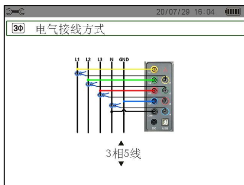
图 5-6 电气连接方式选择
