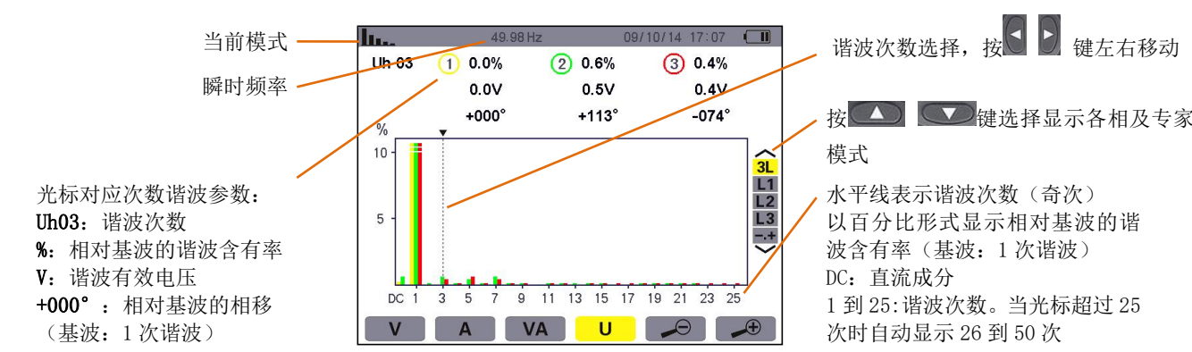
图 7-8 线电压谐波 3L 显示
