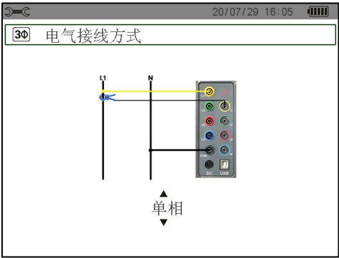
图 4-4 单相连接
