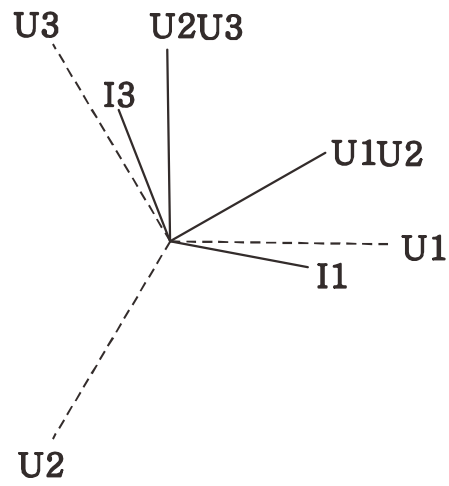
三相三线向量图
