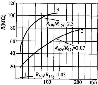
图 1 某台发电机绝缘电阻 R 与时间 t 的关系 极化指数参考判定值：
