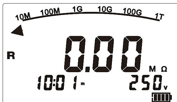
图 9-3 极化指数模式
