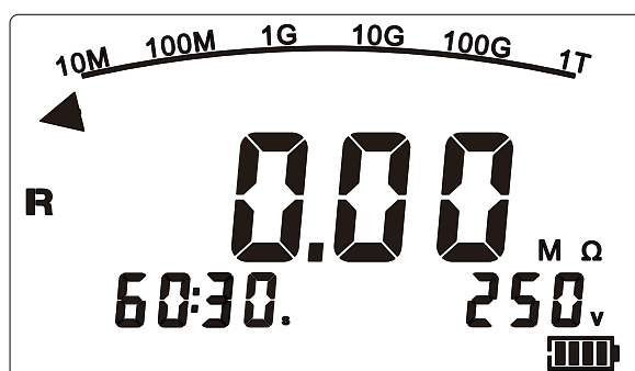
图 9-2 吸收比模式 30 秒模式
